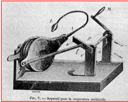
Appareil de Monsieur Gréhant Appareil de Monsieur Vigne
